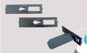
スタビライザーゲージ スタビライザーブレードの取り付け角を合わせるゲージ です。全長が約14cmと長いので、より正確に取り 付けできる。
