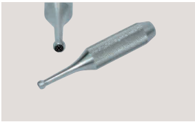
ロッドエンドトリマー ロッドエンドの穴を削ることで、リンクagesをスムーズに することができる工具。先端部のネジで削る量を調整 することが可能。
