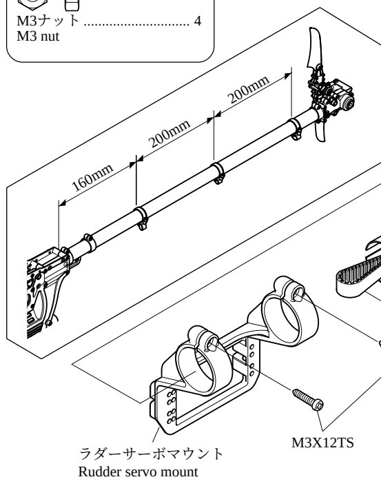
タイミングベルト Timing belt
