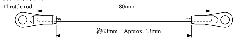
スロットルロッド
