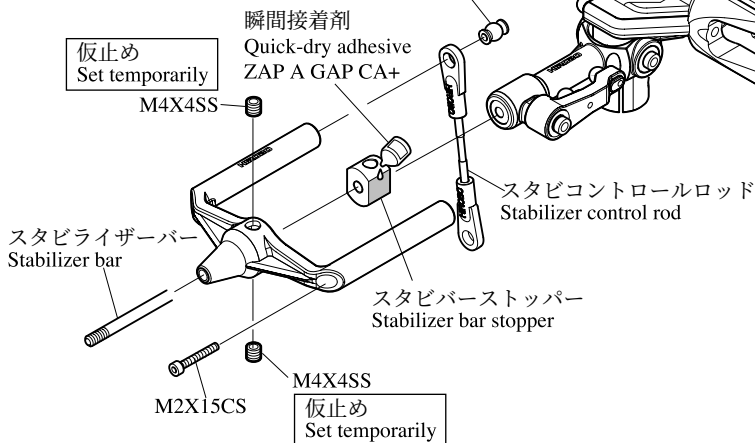
スタビコントロールロッド (2set) Stabilizer control rod
