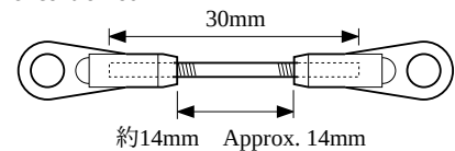
スタビコントロールロッド (2set) Stabilizer control rod
