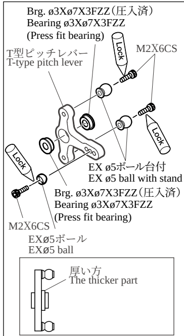
コレクティブピッチロッド Collective pitch rod
