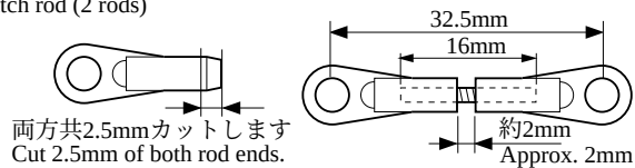
ピッチロッド(2セット) Pitch rod (2 rods)
