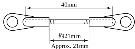
コレクティブピッチレバー/T型レバーロッド Collective pitch lever/T-type lever rod
