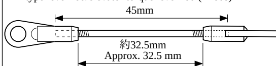
X型レバー / エレベータートルクレバーロッド (2セット) X-type lever rod/elevator torque lever rod (2 rods)
