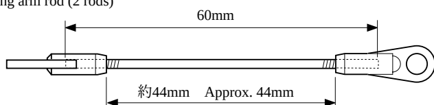
ミキシングアームロッド(2セット) Mixing arm rod (2 rods)
