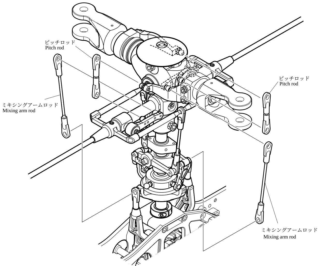
M2ロッドエンド ..... 8 M2 rod end
