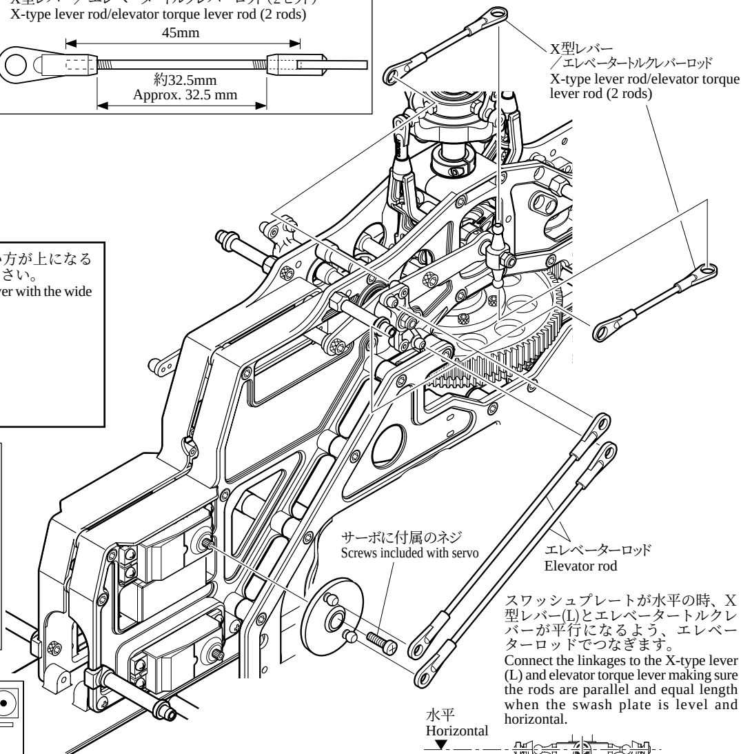
X型レバー / エレベータートルクレバーロッド (2セット) X-type lever rod/elevator torque lever rod (2 rods)
