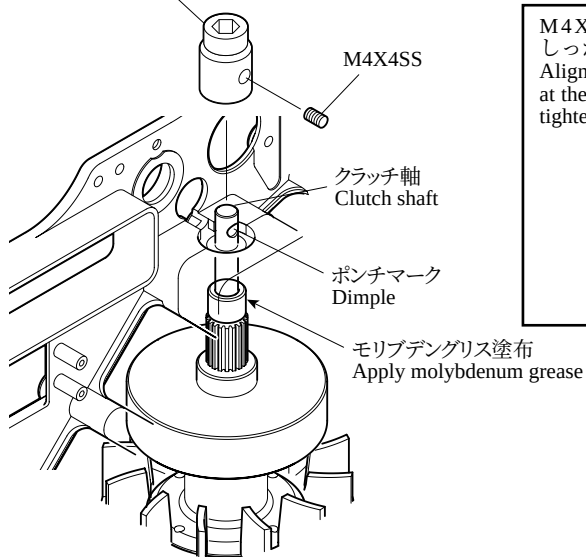
スターターカップリング Starter coupling
